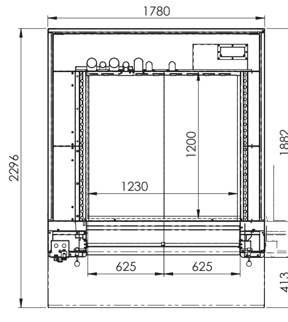
SEZIONE B-B
