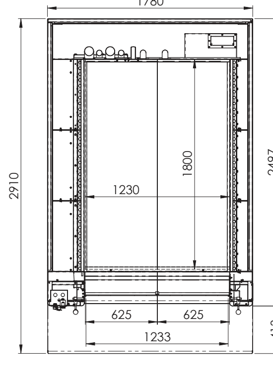
SEZIONE B-B
